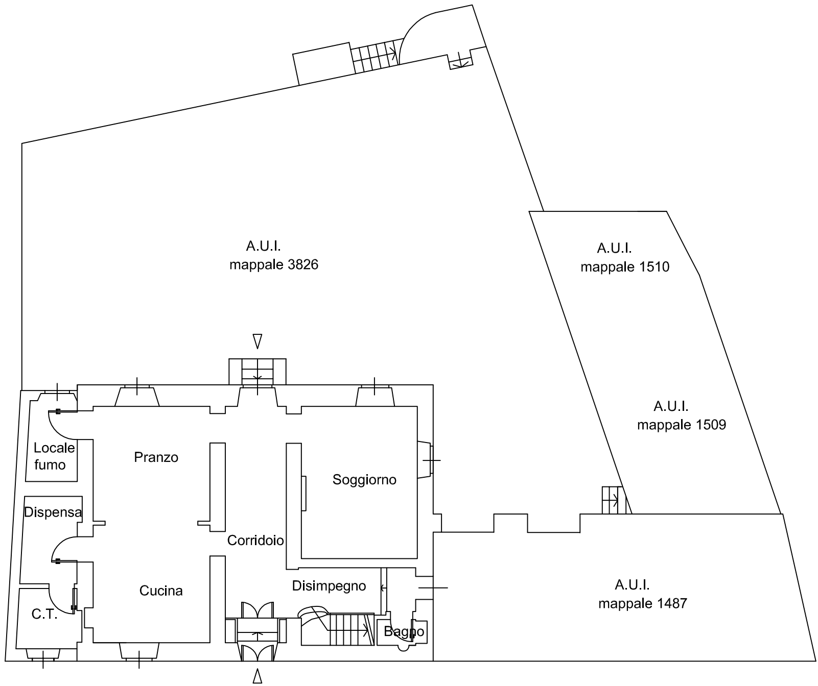
PIANO TERRA (h. 3,70 m)
