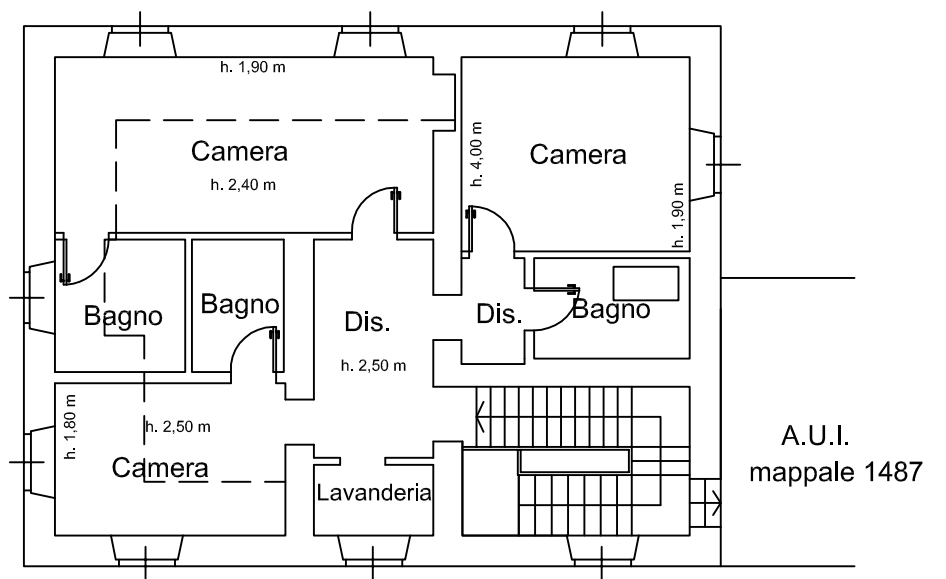
PIANO SECONDO (SOTTOTETTO)
