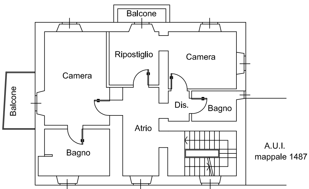
PIANO TERRA (h. 3,70 m)
